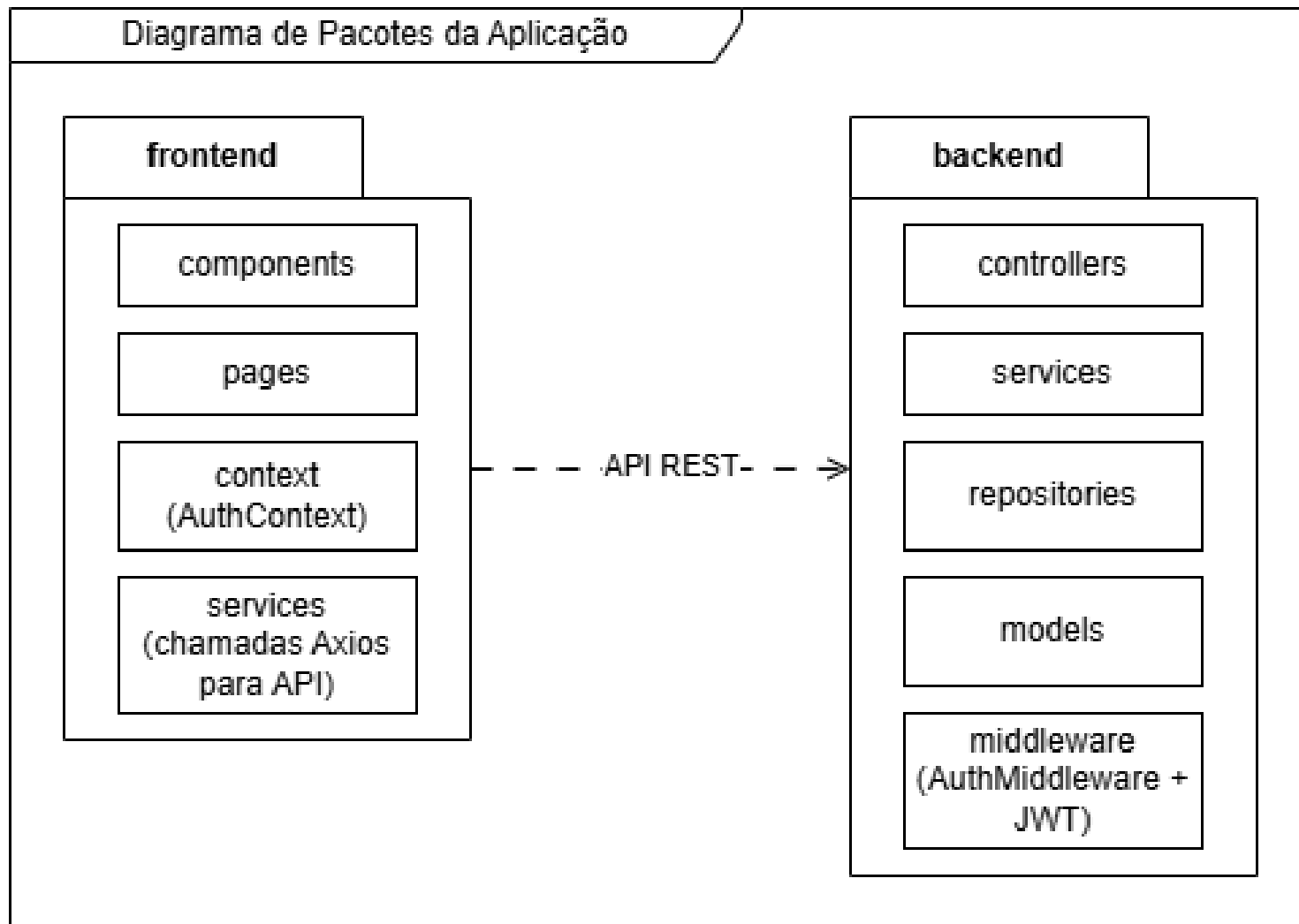
Figura 16: Diagrama de Pacotes da Aplicação
