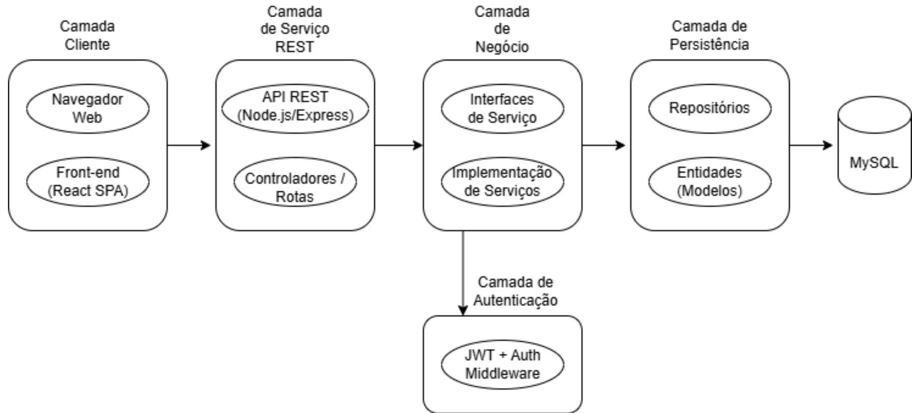
Figura 15: Diagrama de Camadas da Aplicação
