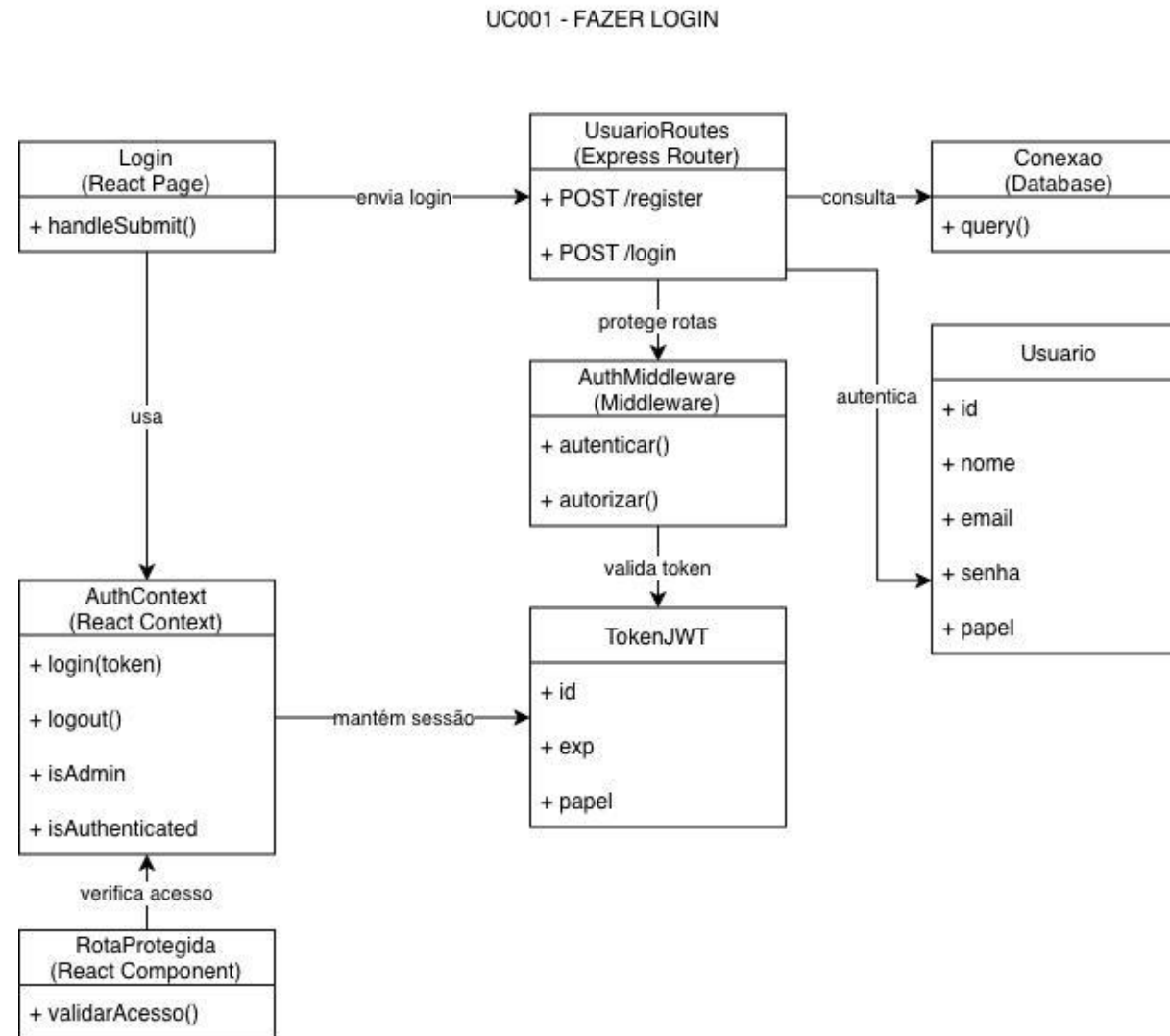
Figura 18: Diagrama de Classes – UC001 Fazer Login
