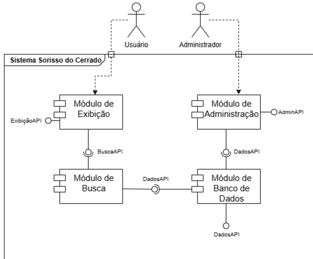
Figura 20: Diagrama de Componentes
