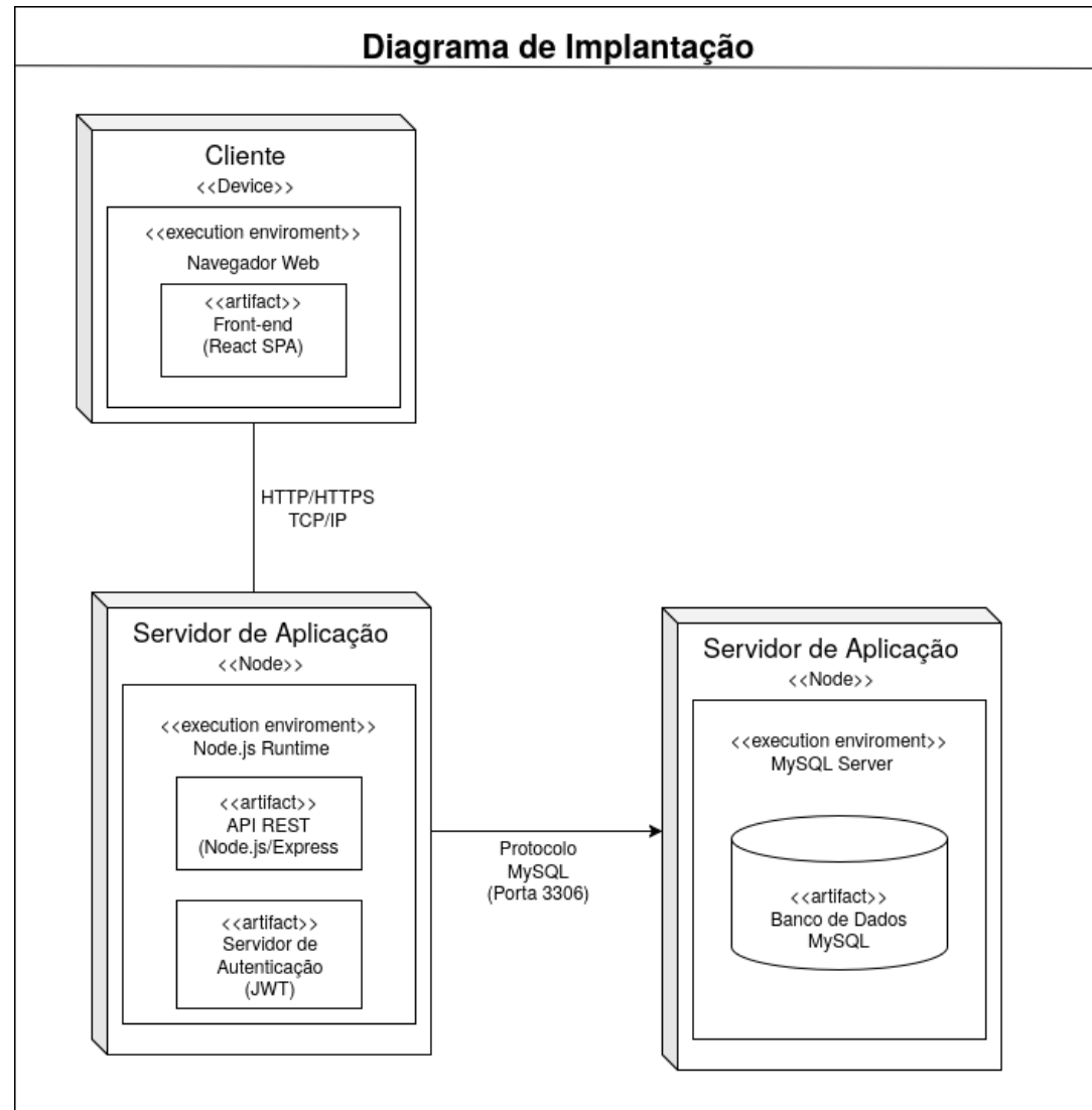
Figura 17: Diagrama de Implantação
