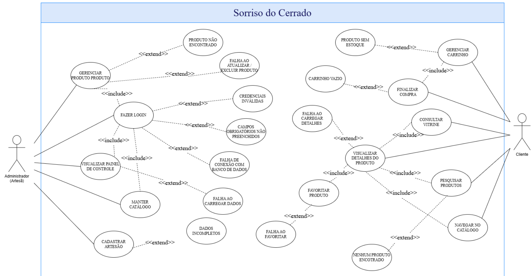
Figura 1: Diagrama de Casos de Uso Geral
