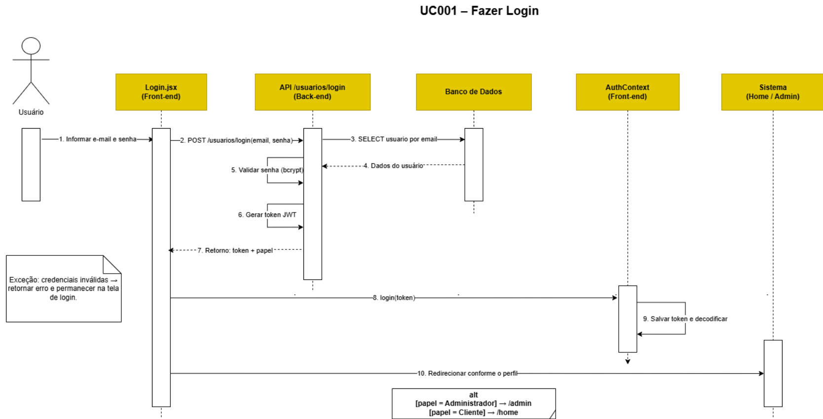
Figura 19: Diagrama de Sequência – UC001 Fazer Login
