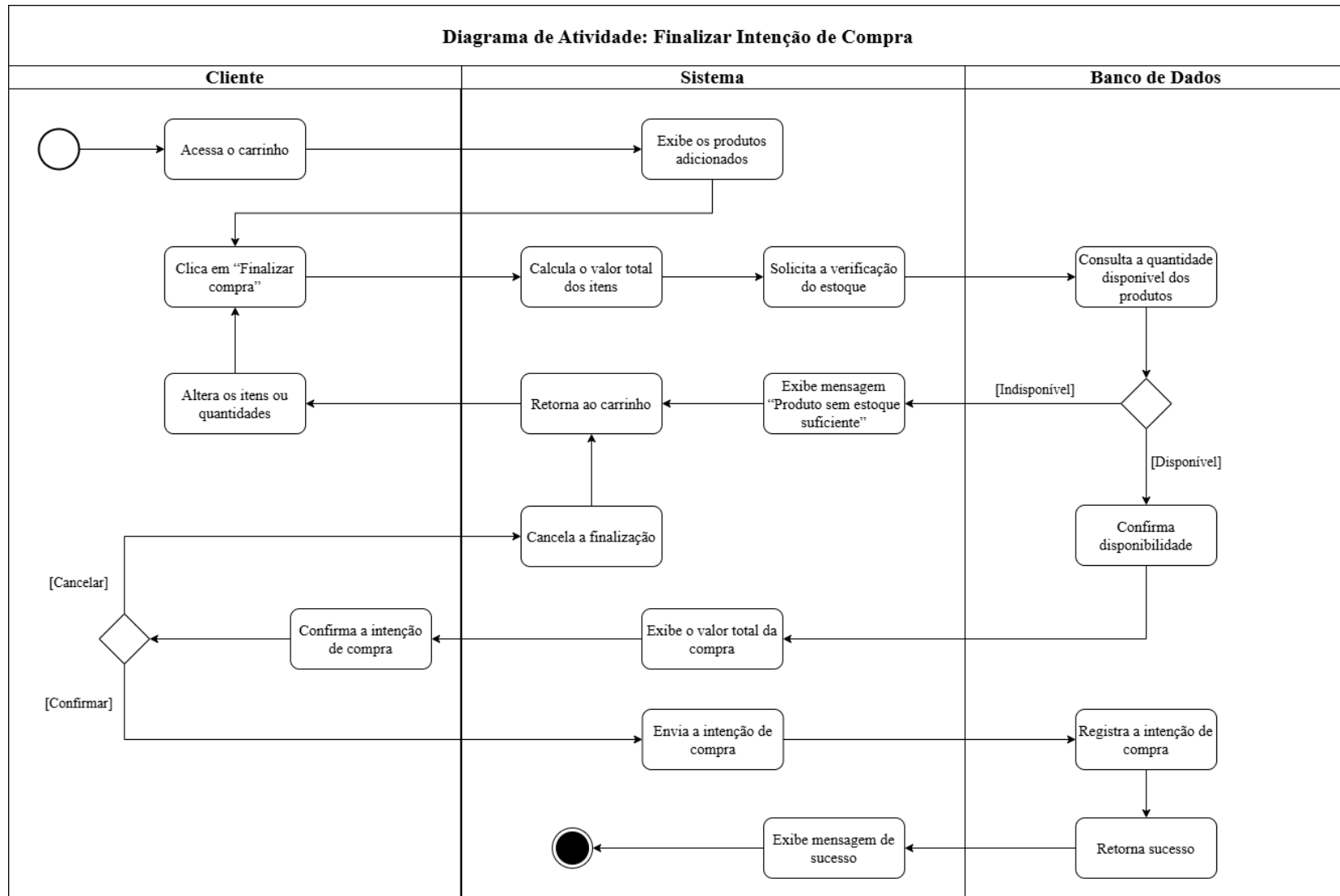
Figura 11: Diagrama de Atividades – Finalizar Intenção de Compra
