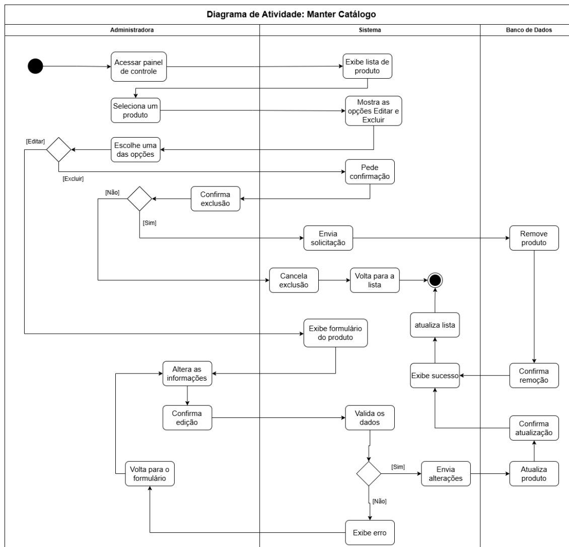
Figura 14: Diagrama de Atividades – Manter Catálogo
