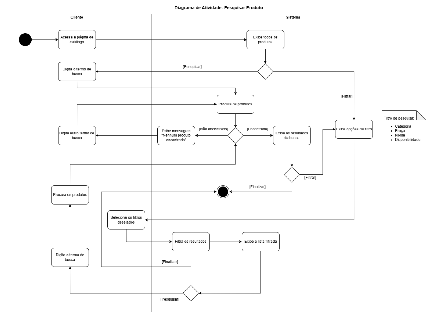
Figura 9: Diagrama de Atividades – Pesquisar Produto
