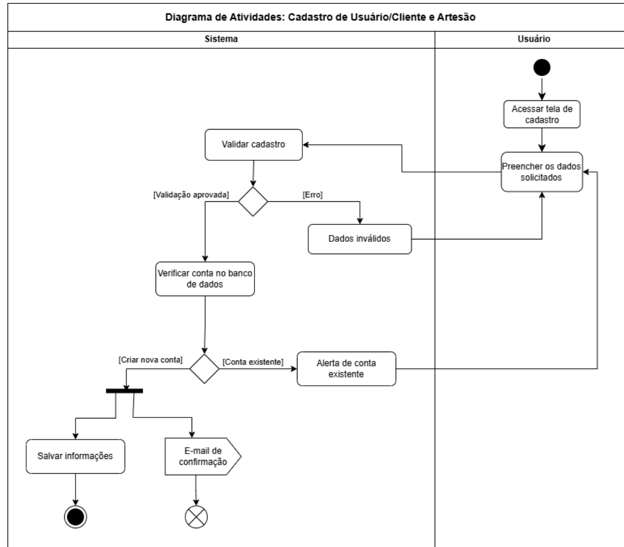
Figura 7: Diagrama de Atividades – Cadastro de Cliente e Artesão
