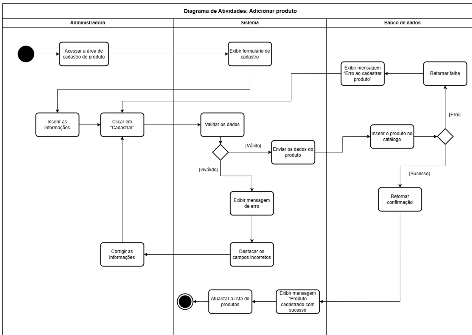
Figura 12: Diagrama de Atividades – Adicionar Produto
