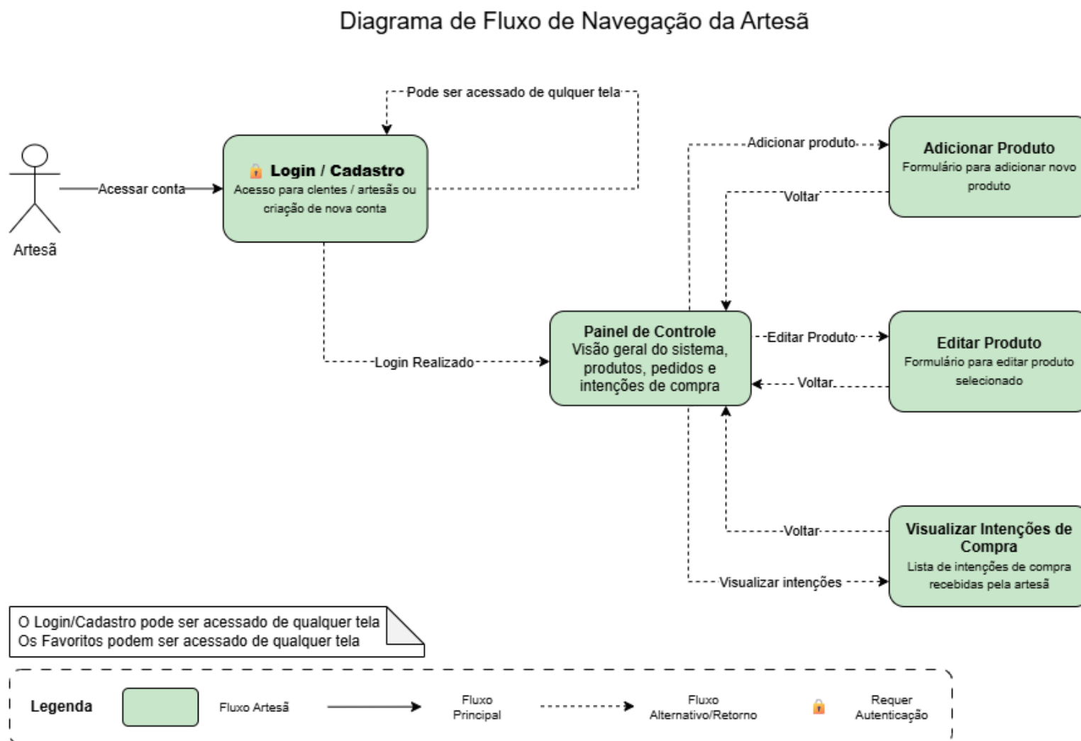
Figura 4: Diagrama de Fluxo de Navegação da Artesã (Administradora)
