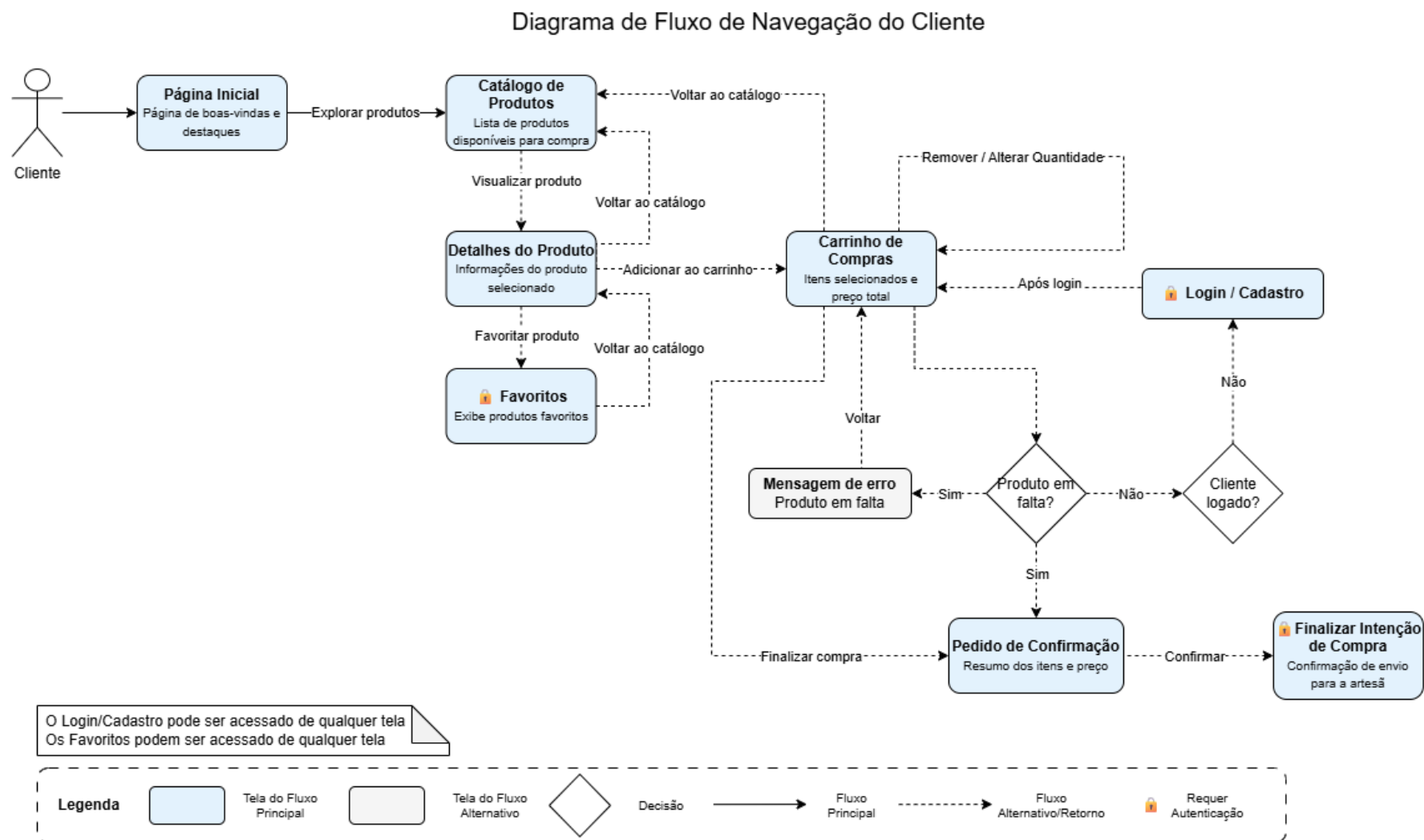
Figura 3: Diagrama de Fluxo de Navegação do Cliente
