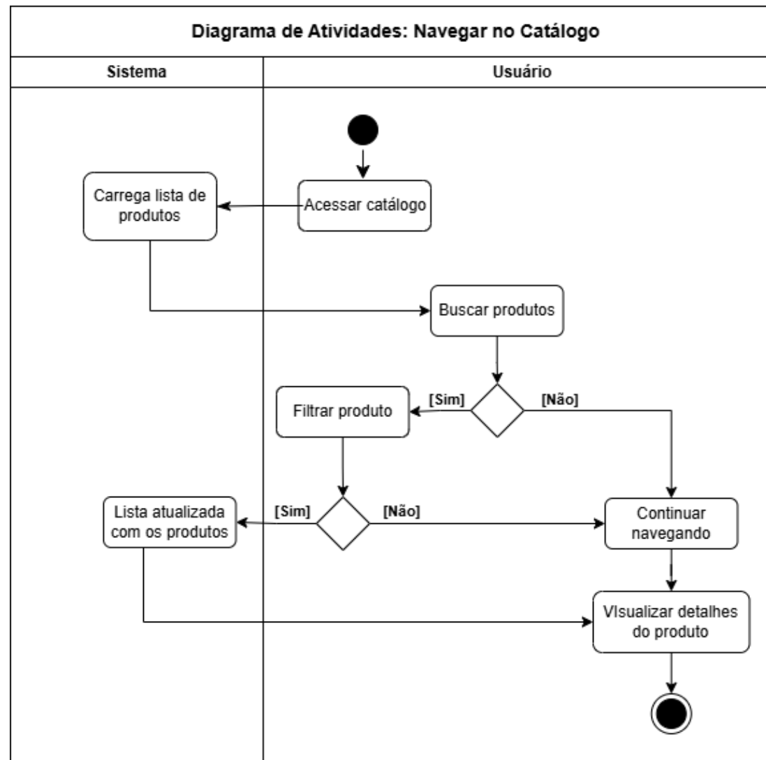
Figura 8: Diagrama de Atividades – Navegar no Catálogo
