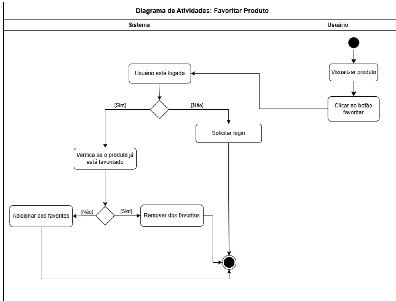
Figura 13: Diagrama de Atividades – Favoritar Produto
