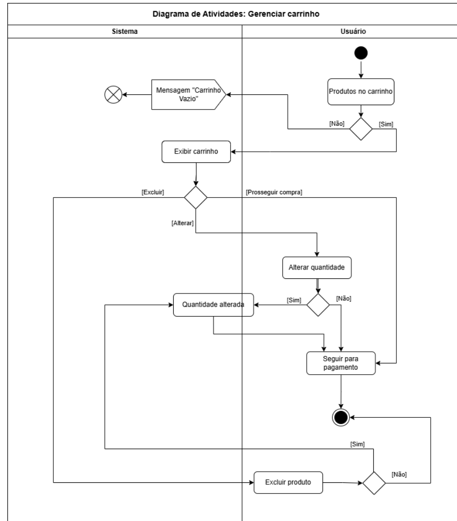
Figura 10: Diagrama de Atividades – Gerenciar Carrinho
