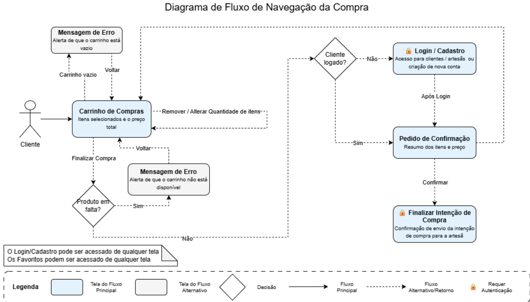
Figura 5: Diagrama de Fluxo de Navegação da Compra (Finalizar Intenção de Compra)
